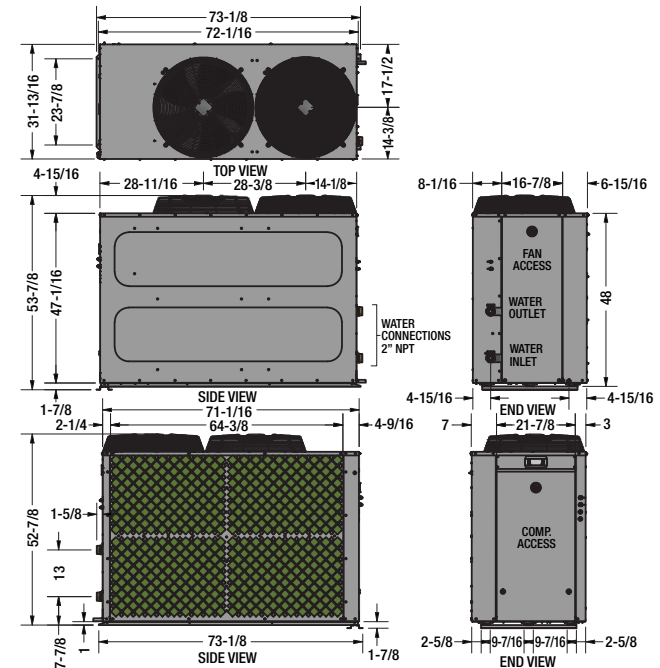
HPHD-135VNU-483 (Vertical)
